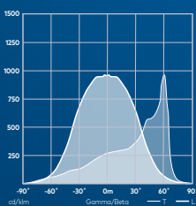
A6 : Optique asymétrique à 60°
