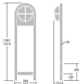
Sloupek pro malou a velkou verzi
